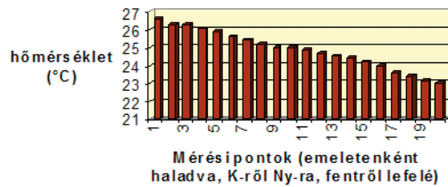
Hőmérsékletváltozása az épületen belüli elhelyezkedés függvényében (fűtési időszakban)
